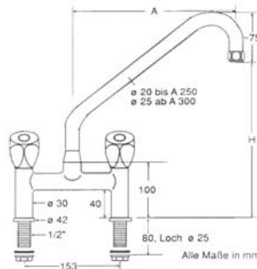
Zweilochbatterie 1/2" schweres Modell, mit Schwenkauslauf 360°, Edelstahlventilsitz, Metallgriff.
