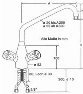
Einlochbatterie 1/2" schweres Modell, mit Schwenkauslauf 360°, Edelstahlventilsitz, Metallgriff.
