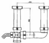
Ablaufverbindung 2" 2 Verstellrohre 2" x 40 x 200 mm, aus Kunststoff weiß, Ausführung 5B.
