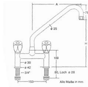
Zweilochbatterie 3/4" schweres Modell, mit Schwenkauslauf 360°, Edelstahlventilsitz, Metallgriff.
